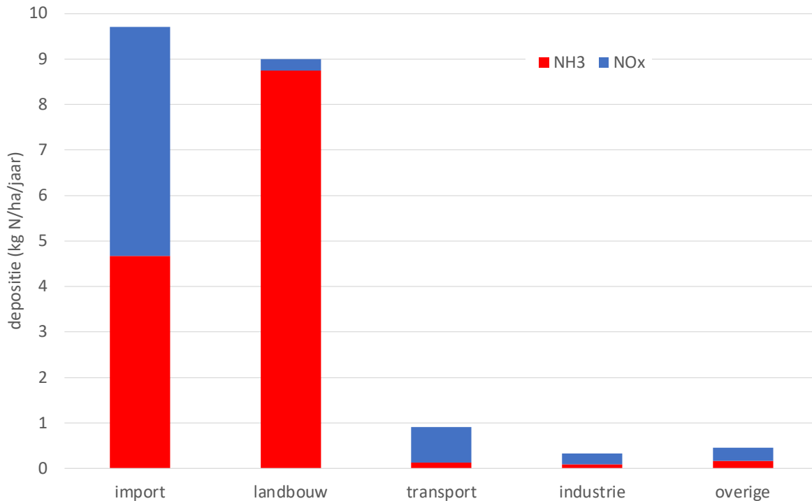
Afb. 3. Bijdragen aan de NH 3 - en NO x -stikstofdepositie (kg N/ha/jaar) door import en de verschillende sectoren in Vlaanderen (2021), gebaseerd op de gegevens van de Vlaamse Milieumaatschappij (VMM; https://www.vmm.be/lucht/stikstof )
